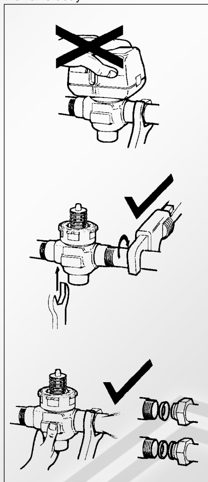
Fig. 11. Plumbing
