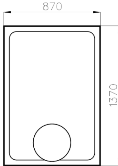
Draufsicht
